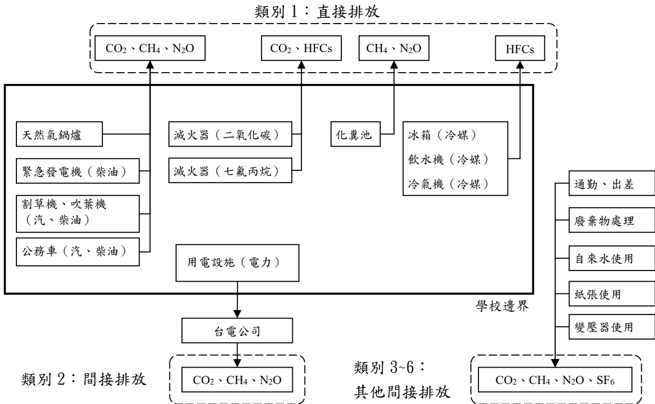
圖4、國立虎尾科技大學組織邊界
